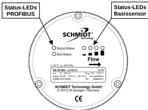
Abbildung 3: Moduldeckel
