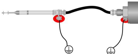
Abbildung 5-1 Erdungsanschlüsse (rot) bei abgesetzter Variante
