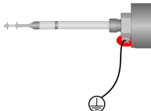
Abbildung 5-2 Erdungsanschluss (rot) bei Kompaktfühler
