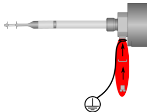
Abbildung 5-1 Erdungsanschlüsse (rot) bei abgesetzter Variante
